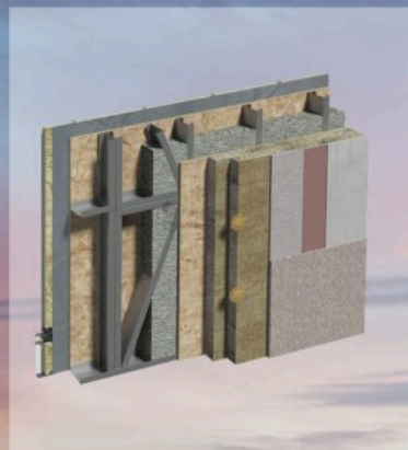
DETALIU FATADĂ
