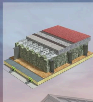
DETALIU PLANSEU
