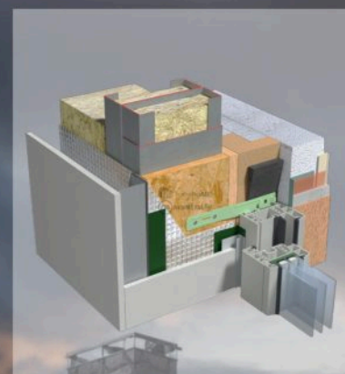
DETALIU TAMPLARIE
