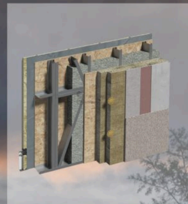
DETALIU FATADĂ
