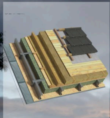
DETALIU ACOPERIS
