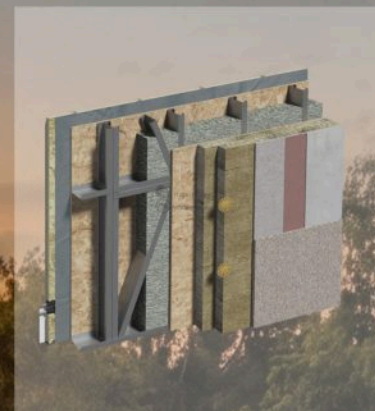
DETALIU FATADĂ
