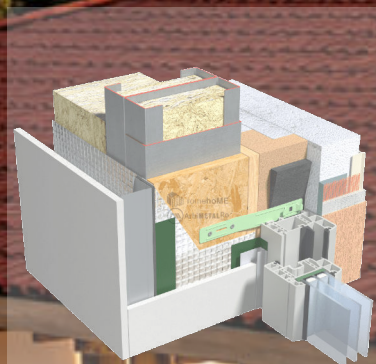
DETALIU TÂMPĂRIE
