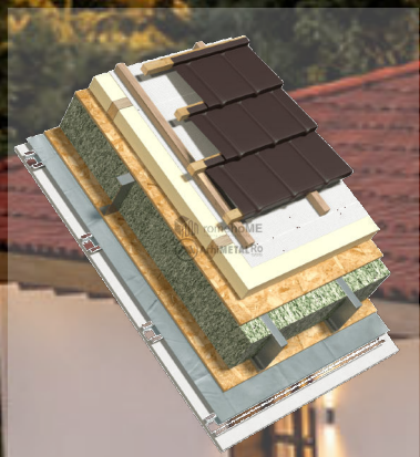
DETALIU ACOPERIȘ
