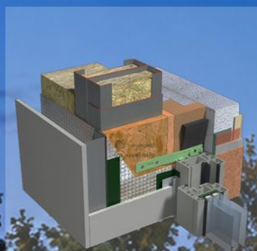
DETALIU TAMPLARIE
