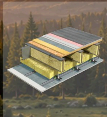
DETALIU PLANȘEU
