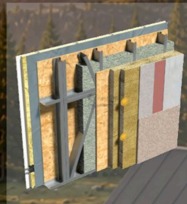
DETALIU FAȚADĂ
