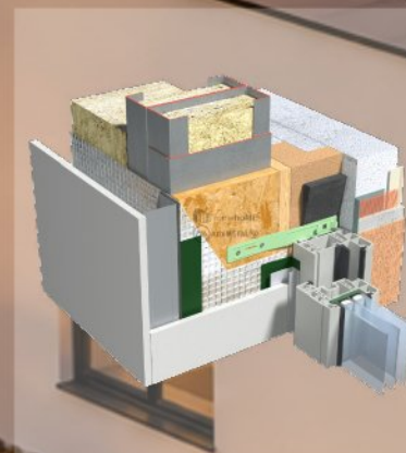
DETALIU TÂMLĂRIE
