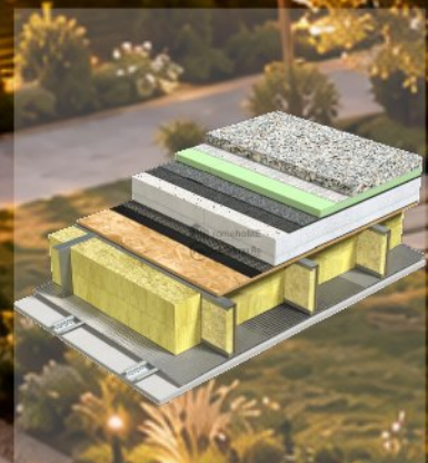
DETALIU TERASĂ
