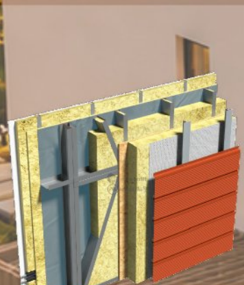
DETALIU FAȚADĂ
