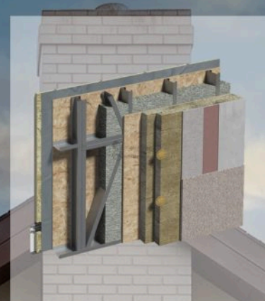
DETALIU FATADĂ
