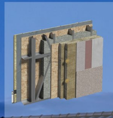
DETALIU FATADĂ
