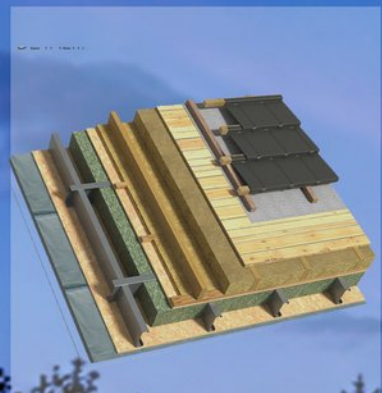
DETALIU ACOPERIS
