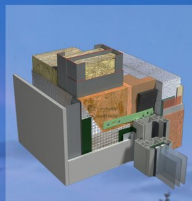
DETALIU TAMPLARIE
