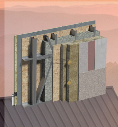
DETALIU FATADĂ
