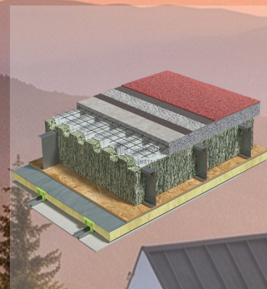
DETALIU PLANSEU
