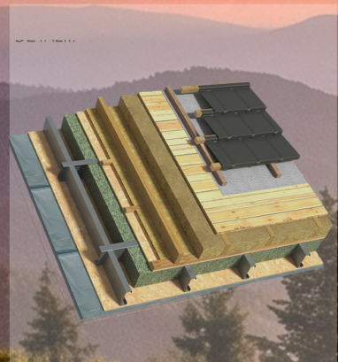
DETALIU ACOPERIS
