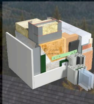
DETALIU TÂMLĂRIE
