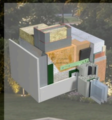
DETALIU TAMPLARIE
