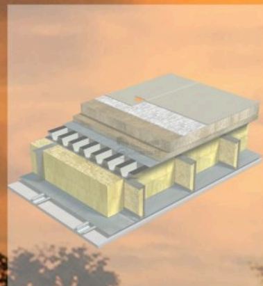
DETALIU TERASA
