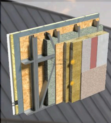
DETALIU FAȚADĂ
