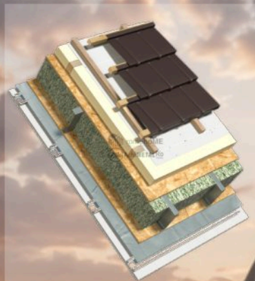
DETALIU ACOPERIȘ
