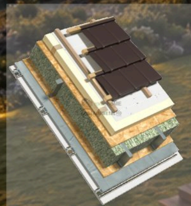
DETALIU ACOPERIȘ
