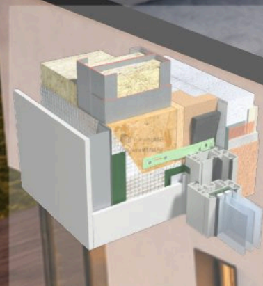
DETALIU TÂMPĂRIE
