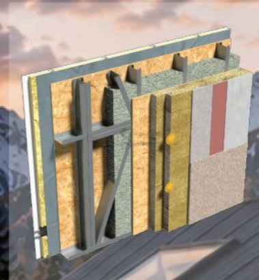
DETALIU FAȚADĂ
