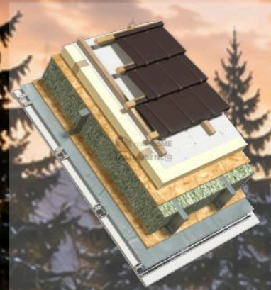
DETALIU ACOPERIȘ
