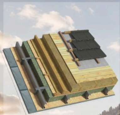
DETALIU ACOPERIS
