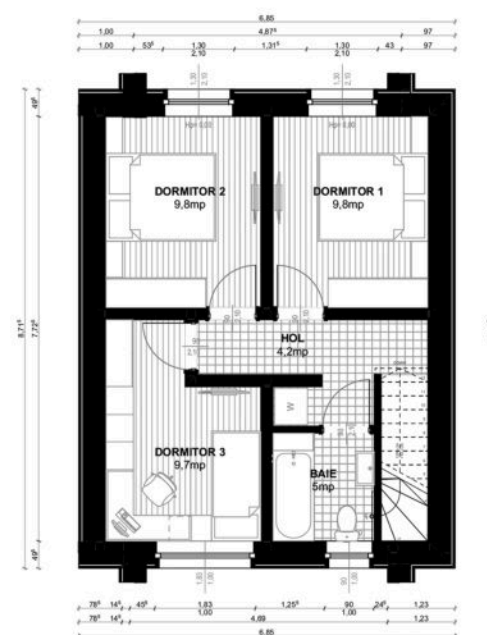
PLAN ETAJ
