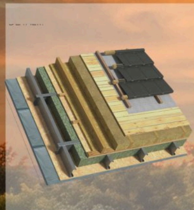
DETALIU ACOPERIS
