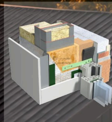
DETALIU TÂMLĂRIE
