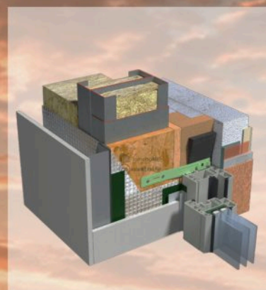
DETALIU TAMPLARIE
