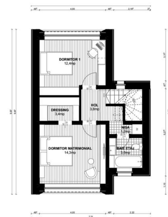
PLAN ETAJ
