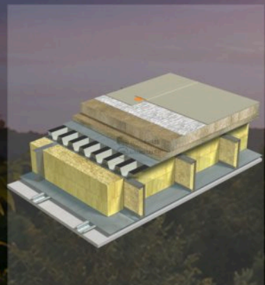
DETALIU TERASA
