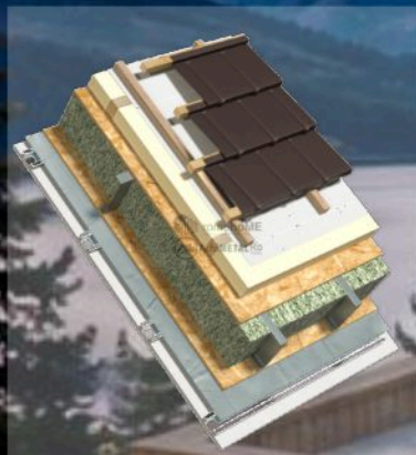
DETALIU ACOPERIȘ
