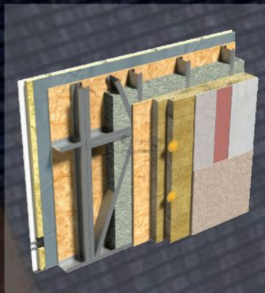
DETALIU FAȚADĂ
